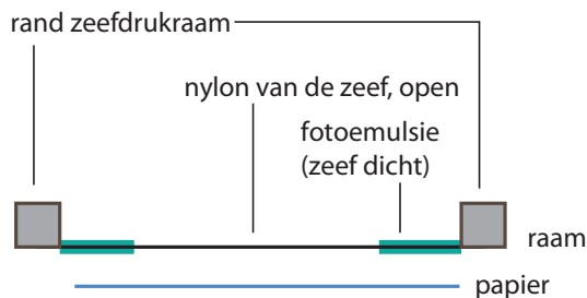
doorsnede zeef met kader
