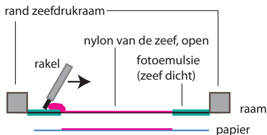
doorsnede, afdrukken met zeef met kader
